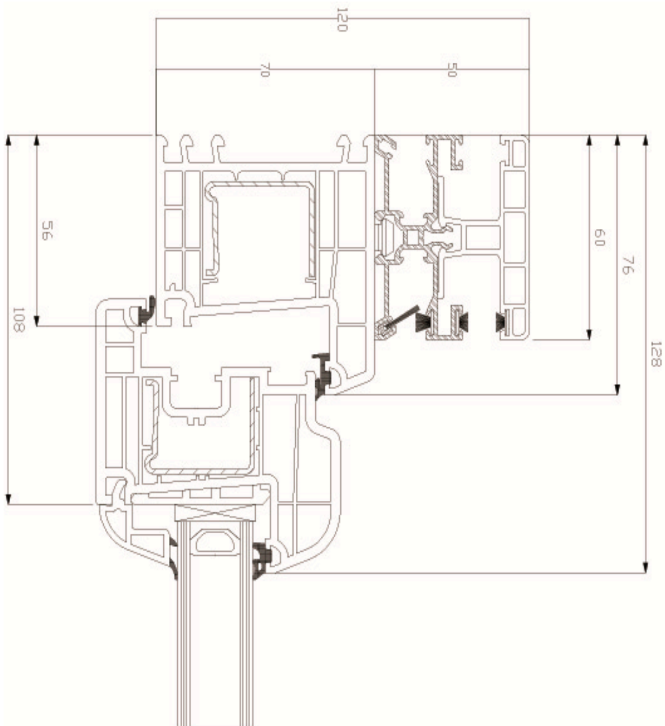
Sección guía de 50mm para mosquitera con marco de 70mm. Serie 799
